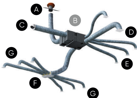
Exemple de schéma de principe des réseaux avec une centrale PRIMOCOSY HR BP
