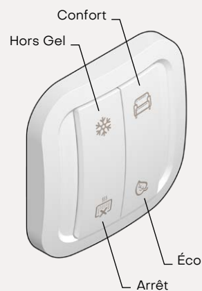
Interrupteur Chauffage Fil Pilote CWS-2-FP-01
