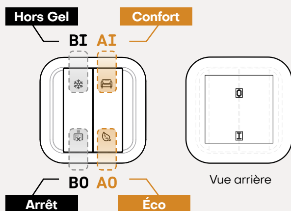
Interrupteur Chauffage Fil Pilote CWS-2-FP-01
